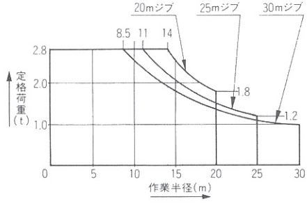
● 定格荷重曲線
