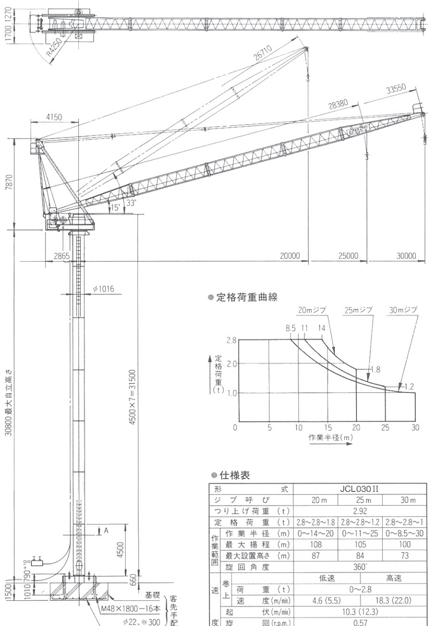
● 寸法図
